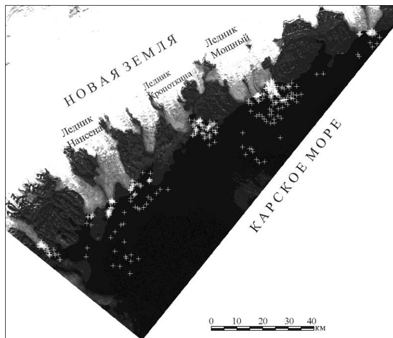
Рис. 3. Пример оперативной информационной продукции об айсбергах Карского моря, подготовленной специалистами ААНИИ для передачи конечному пользователю.
