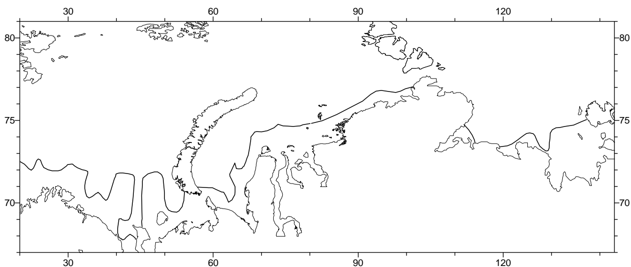
Рис. 1. Южная граница распространения в Баренцевом и Карском морях по данным ледовых авиаразведок за период 1928-1991 гг. [Abramov, 1996; Ледяные, 2006].
