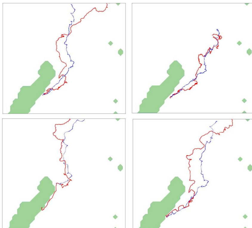
Рис. 4. Сопоставление наблюдаемых (красная) и рассчитанных по модели (синяя) траекторий айсбергов.
