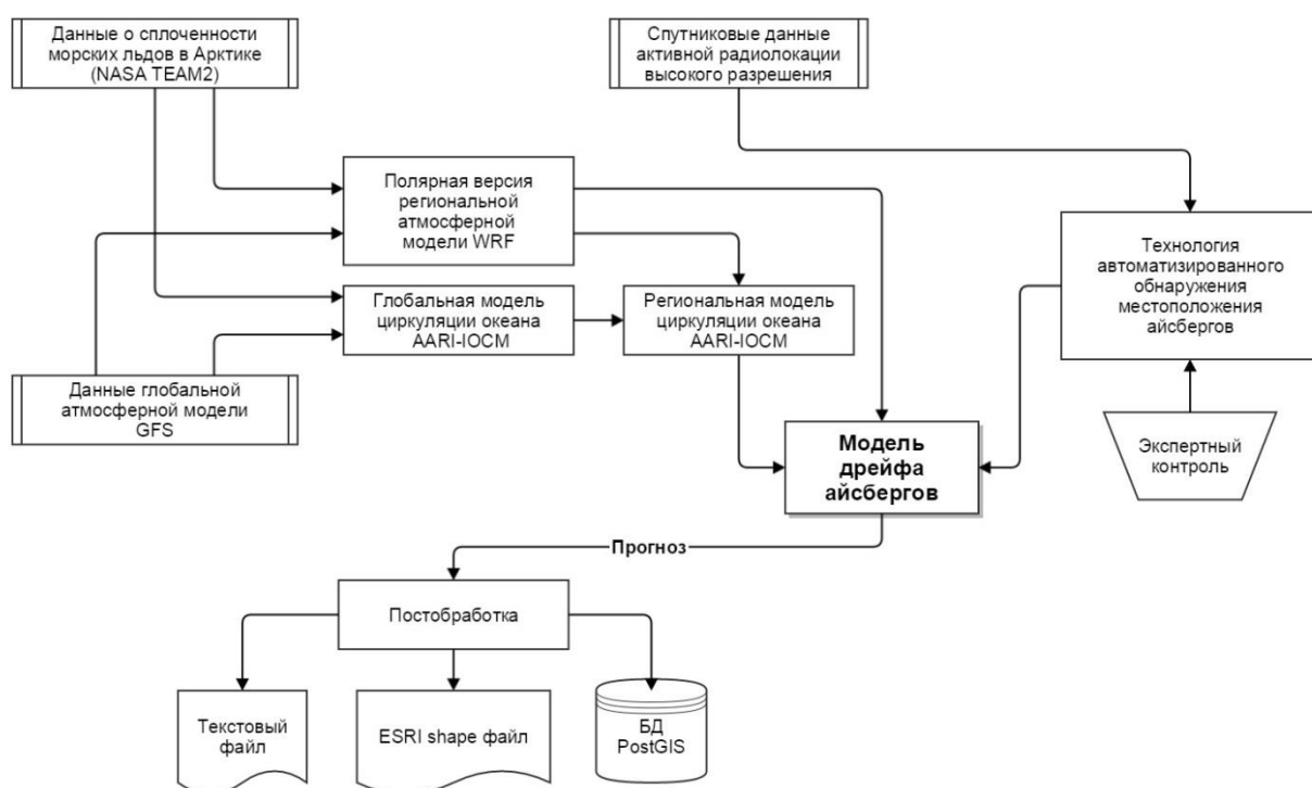
Рис. 5. Схема технологии прогноза дрейфа айсбергов.
